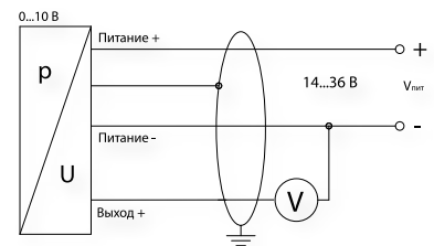
3-проводное исполнение: 0...10 V
