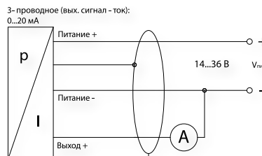
3-проводное исполнение: 0...20 mA
