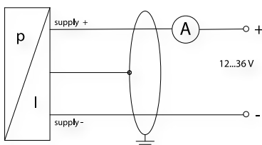
2-проводное исполнение: 4...20 mA
