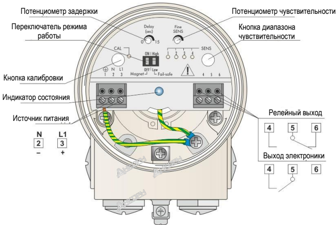
Варианты подключения реле и выхода электроники
