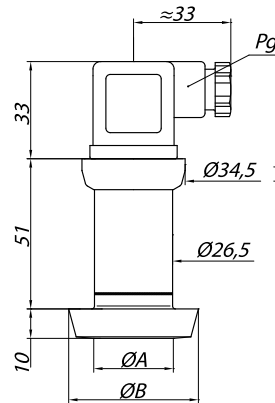
Торцевая мембрана
