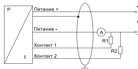
2-х проводная схема с двумя дискретными выходами
