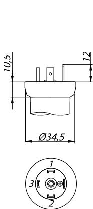
DIN 43650
