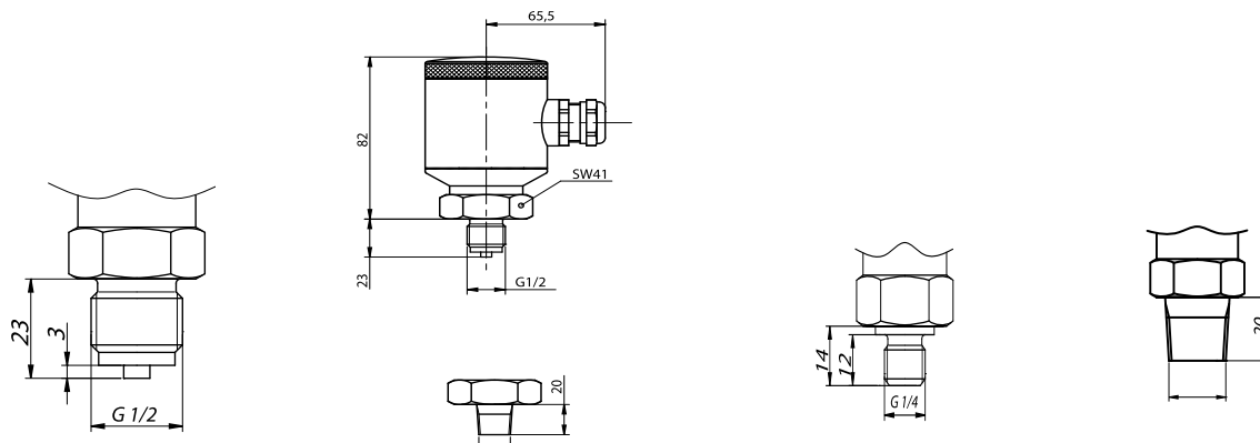
G 1/2" EN 837
