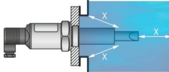
Модель с фланцем, предельное расстояние x > 5 мм
